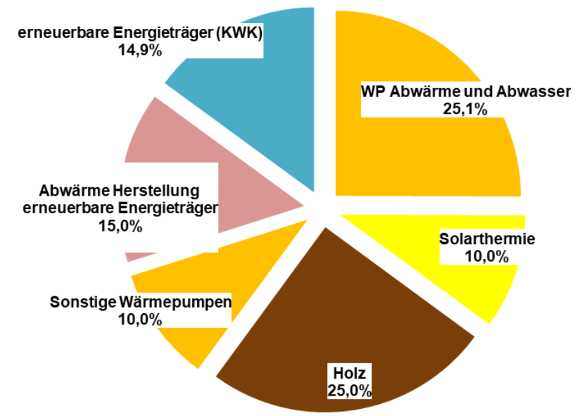
Abb. 45: mögliche Wärmeerzeugung Zielfoto Fernwärme 2040
